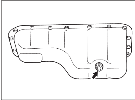
Ροπή σύσφιξης τάπας αποστράγγισης 35 Nm (3.6 kg-m, 25.8 lb-ft)
