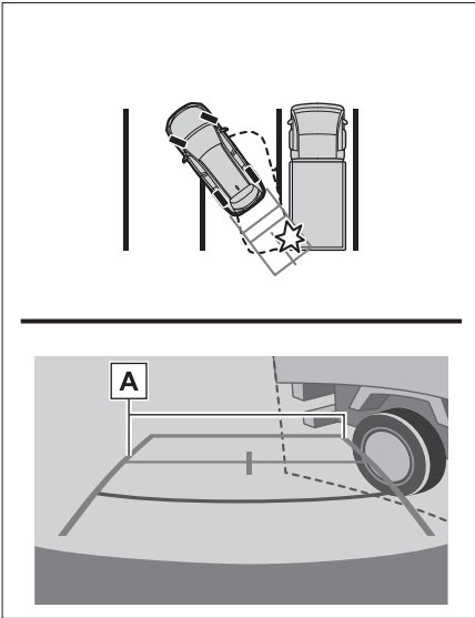
A Γραμμές-οδηγοί πλάτους αυτοκινήτου
