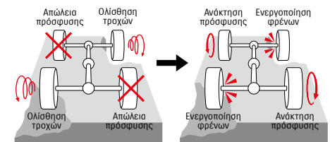
Χωρίς brake LSD Με brake LSD
